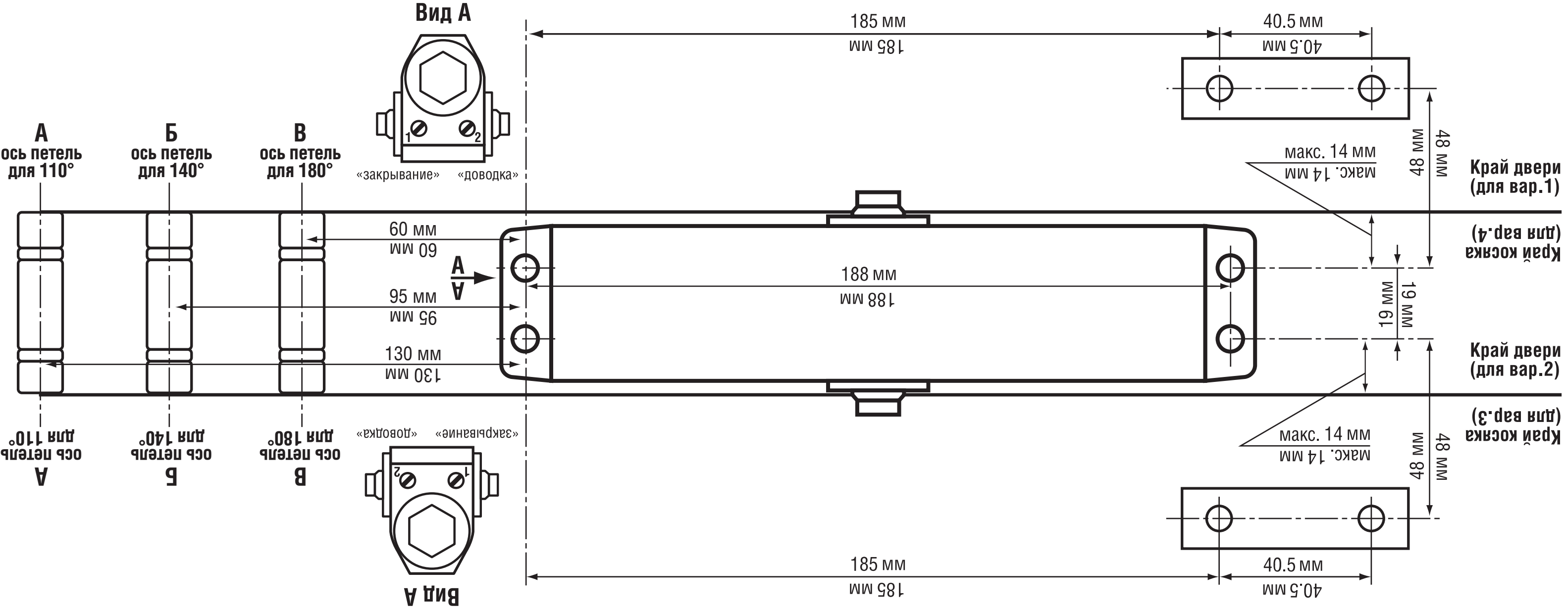
Стандартная установка для левой двери
